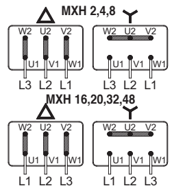
Schema elettrico Electrical diagram Schaltbild Schéma électrique Esquema eléctrico 电气图
