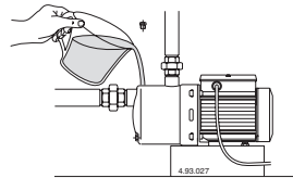
Fig. 4 Riempimento Filling Auffüllung Remplissage Llenado 灌泵
