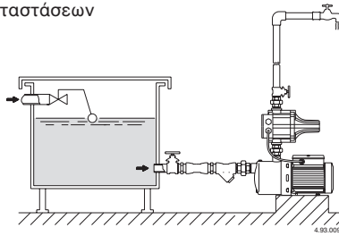
Fig. 1 Funzionamento sotto battente Positive suction head operation Zulaufbetrieb Fonctionnement en charge Funcionamiento bajo carga 正压上水头的操作
