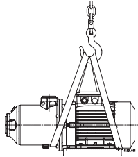
Sollevario pompa Raising the pump Anhebung Pumpe Suollevamento de la pompe Elevación de la bomba 吊起水泵
