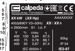
Esempio targhetta motore
