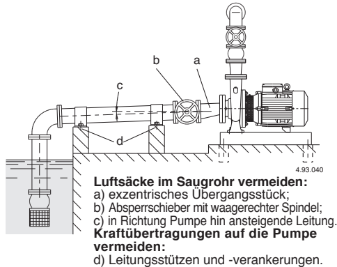
Abb. 2 Anschluß der Rohrleitung.
